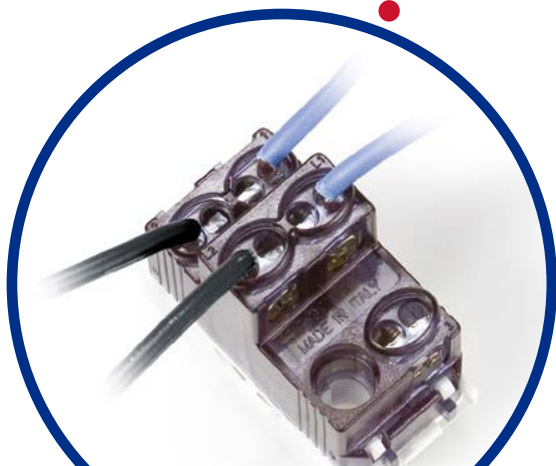
UTILIZZO INTERRUTTORE 2P
