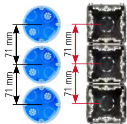
3 scatole tonde 00402/00411 o quadrate 00418 in verticale
