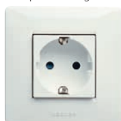
blanc M21176 ivoire M22176 Prise Schuko 2P+E 16A, norme allemande
